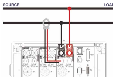
外部电流互感器接线
