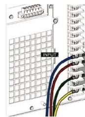
交流三相输入(Y接法)
