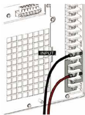
交流单相输入
