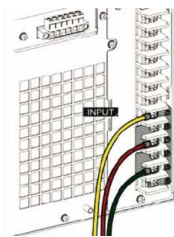
交流三相输入(Δ接法)
